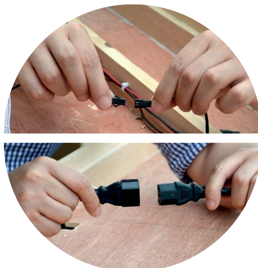
Prepojenie káblov
